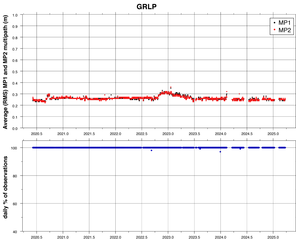
Figura 4.3: Analisi di qualità per ciascuna misura gionalliera della stazione GRLP in termini di multipath MP1 in nero e MP2 in rosso (sopra), e di percentuale di osservazioni presenti nei RINEX giornalieri rispetto alle osservazioni attese nell'intervallo di tempo gionalliero di funzionamento effettivo (sotto).
