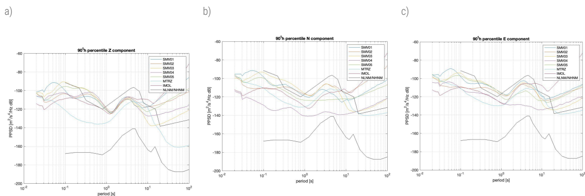
Figura 2.2. Curve di rumore calcolate dal 90° percentile delle PPSP del mese di Febbraio 2024 per tutte le stazioni della rete integrata alle tre componenti Z, N e E rispettivamente da sinistra a destra. Le linee nere indicano l'andamento dei valori di rumore minimo NLNM (New Low Noise Model) e massimo NHNM (New High Noise Model) definiti da Peterson (1993) come riferimento.
